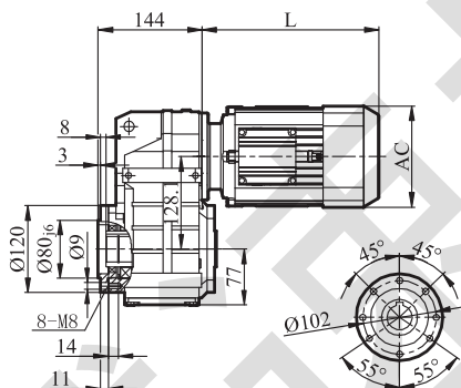
GFAZ/GFHZ/GFVZ47
