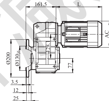
GFH/GFHZ/GFHF47输出轴
