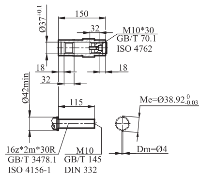
GFV/GFVZ/GFVF47输出轴
