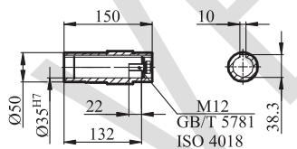
GFA/GFAZ/GFAF47输出轴
