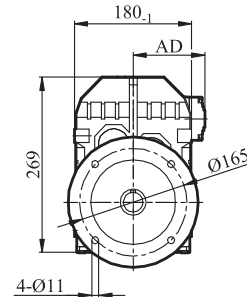
GFV/GFVZ/GFVF47输出轴
