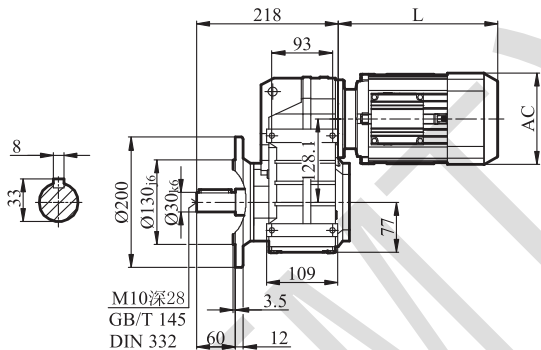
GFA/GFAZ/GFAF47输出轴
