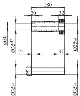
GFH/GFHZ/GFHF47输出轴
